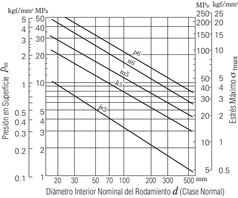
Fig. 15.5 Presión en Superficie P_m y Estrés Máximo \sigma_{\text{max}} para Interferencia de Ajuste Intermedia
