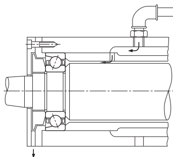
Fig. 12.9 Lubricación por Niebla de Aceite
