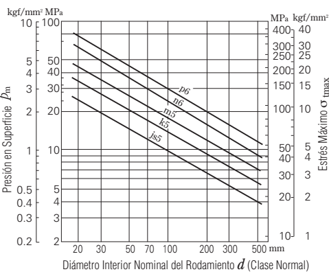
Fig. 15.6 Presión en Superficie P_m y Estrés Máximo \sigma_{\text{max}} para Interferencia de Ajuste Máxima
