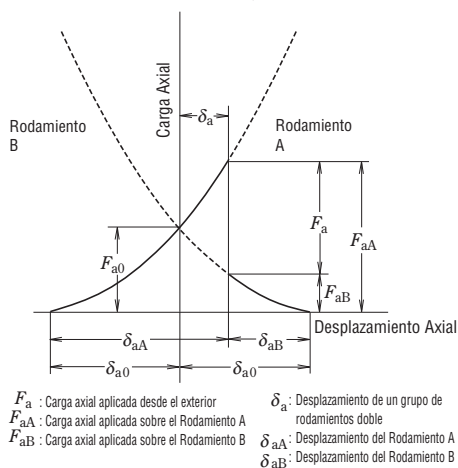
Fig. 10.4 Desplazamiento Axial con Precarga de Posición
