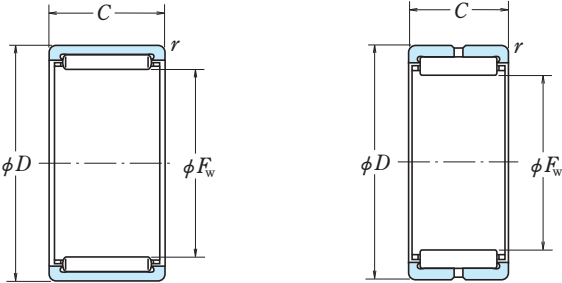
Sin Anillo Interior
